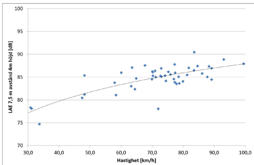
Figur 4 Uppmätt A-vägd ljudexponeringsnivå 7,5 m från fordonsmitt för enskilda fordon i kategori 3.
