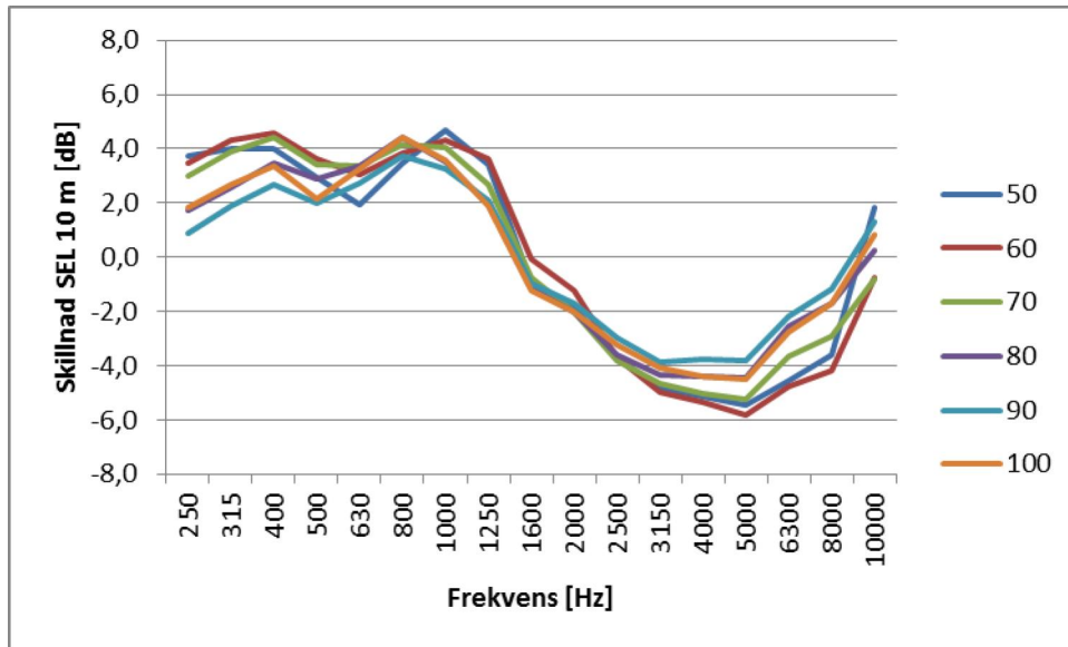
Figur 55 Skillnad mellan uppmätt ljudexponeringsnivå och beräknad med Nord2000 Road på 10 m avstånd och 4 m höjd. Kurvorna förskjutna så att medelvärde är 0. Kategori 1. OBS frekvensrådet.
