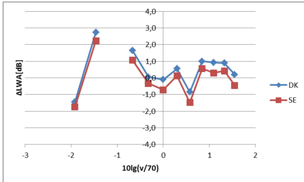
Figur 47 Skillnad i A-vägd ljudeffektnivå mellan mätning och beräkning enligt Nord2000 Road (DK) respektive med svenska korrekationer (SE) för kategori 3 fordon.
