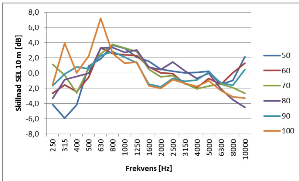
Figur 59 Skillnad mellan uppmätt ljudexponeringsnivå och beräknad med Nord2000 Road på 10 m avstånd och 4 m höjd. Kurvorna förskjutna så att medelvärdet är 0. Kategori 3. OBS frekvensområdet.
