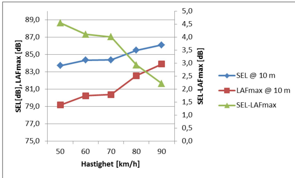
Figur 52 Uppmätta ljudexponeringsnivåer respektive maximalnivåer på 10 m avstånd, samt skillnaden mellan dem som funktion av hastighet. Tunga fordon.
