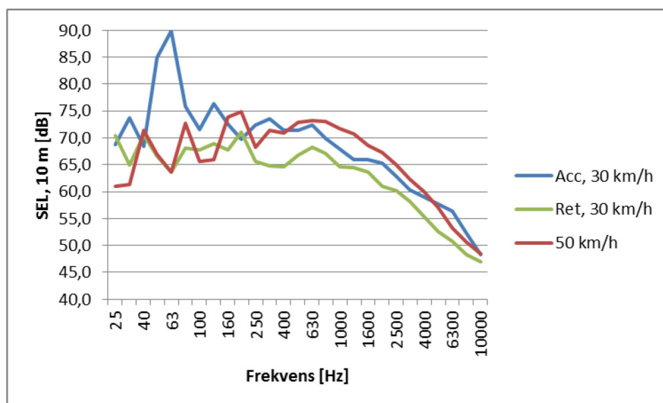
Figur 80 Uppmätt ljudexponeringsnivå på 10 m avstånd 4 m höjd vid busshållplats. Kategori 3 fordon som accelererar, retarderar respektive förbipassager i konstant hastighet.
